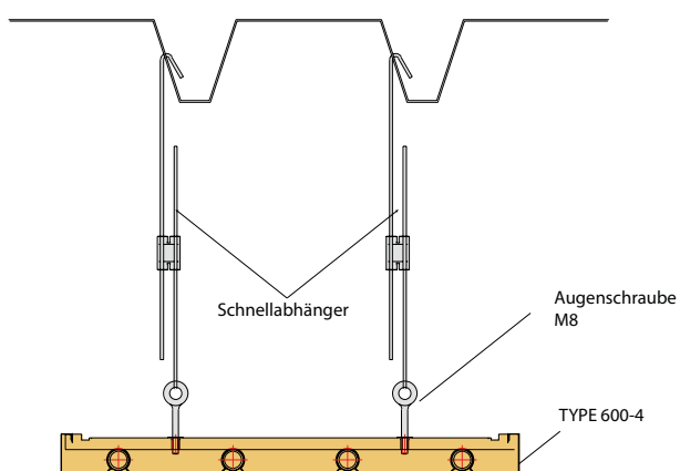
Methode D: Verwendung von Schnellabhängern
