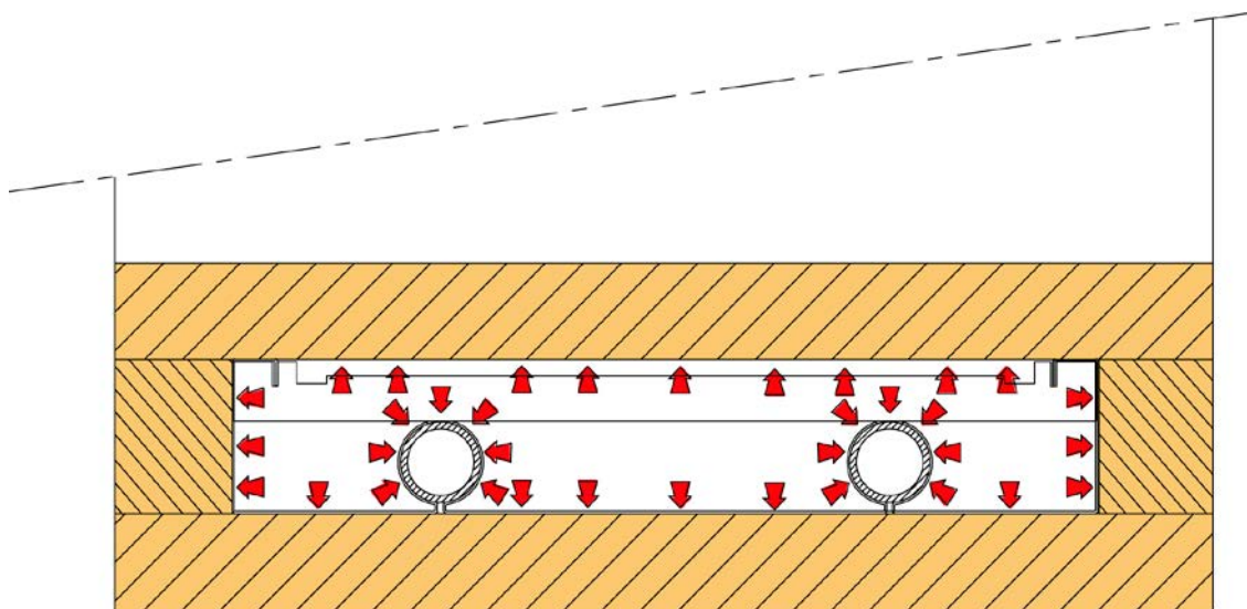
Die Formschablone mit Strahlungspaneel
