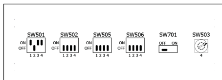
Image 5.5.4 : Position des commutateurs DIP.
