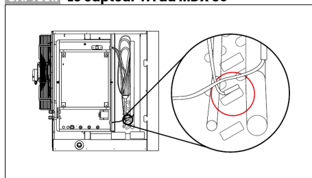
Image 7.5.1.5 : Capteurs TC du Mistral MDX 30.
