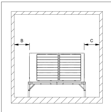
Image 4.2.2.2 : Unité intérieure avec cadre debout.
