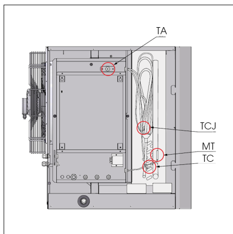
Image 7.5.1.4 : Capteurs du Mistral MDX 30.
