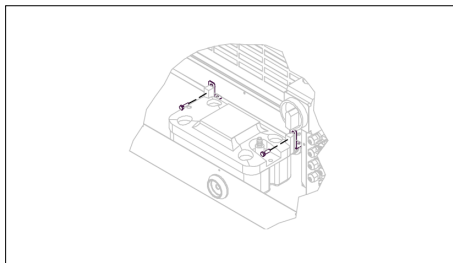
Image 7.5.2.3 : Démonter la pompe à condensats.
