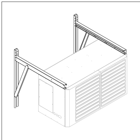
Image 5.2.2.1 : Vue de la méthode de montage.
