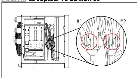
Image 7.5.1.12 : Capteurs TCJ du Mistral MDX 60.
