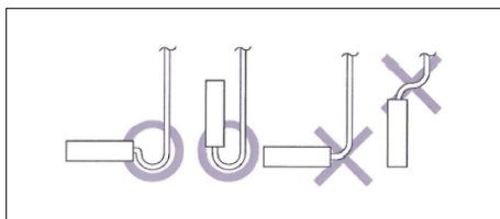
Image 7.5.1.3 : Vue de la position correcte du câble.
