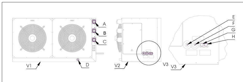
Image 2.1.3.1: Pièces pour l'installation du MISTRAL MDX 60. (V1 : Vue arrière, V2 : Vue latérale gauche)
