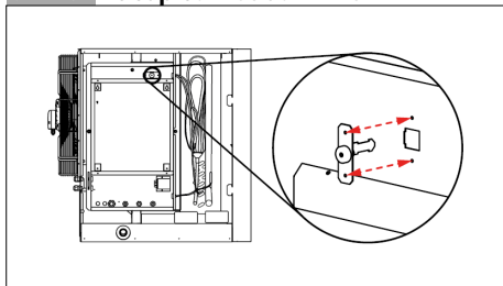
Image 7.5.1.7 : Capteurs TA du Mistral MDX 30.
