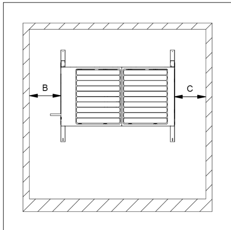
Image 4.2.1.2 : Unité intérieure avec support mural.
