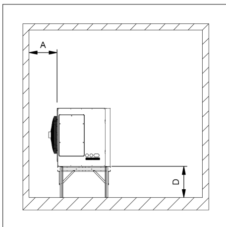
Image 4.2.2.1 : Unité intérieure avec cadre debout.
