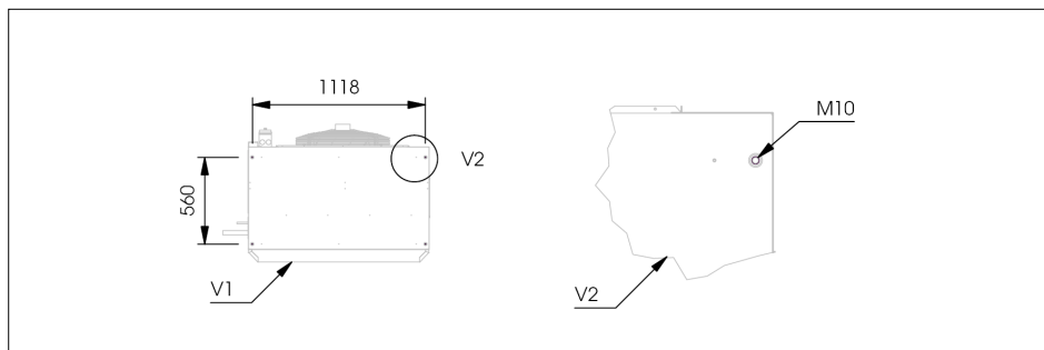
Image 2.1.2.4 : Points de suspension du MISTRAL MDX 30. (V1 : Vue de dessus)
