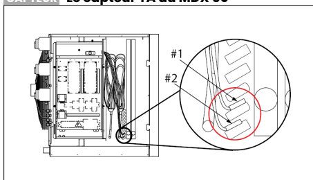
Image 7.5.1.11 : Capteurs TC du Mistral MDX 60.
