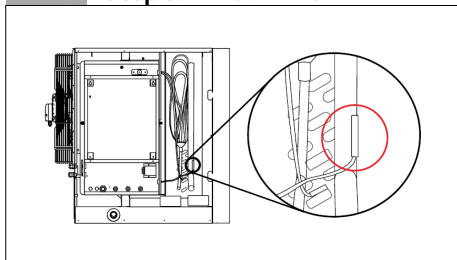
Image 7.5.1.8 : Capteurs MT du Mistral MDX 30.
