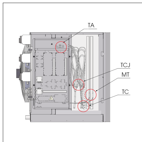
Image 7.5.1.10 : Capteurs du Mistral MDX 60.
