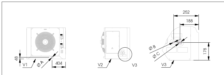
Image 2.1.2.5 : Dimensions des connexions MISTRAL MDX 30. (V1 : Vue arrière, V2 : Vue latérale gauche)
