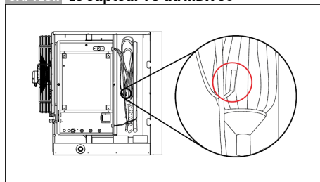
Image 7.5.1.6 : Capteurs TCJ du Mistral MDX 30.
