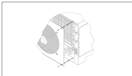
Image 7.5.2.2 : Démonter la paroi du ventilateur.
