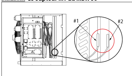
Image 7.5.1.14 : Capteurs MT du Mistral MDX 60.
