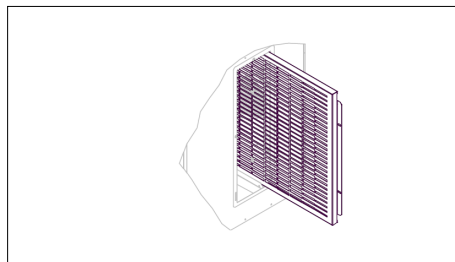
Image 7.4.3.2 : Retrait de la plaque de distribution d'air.
