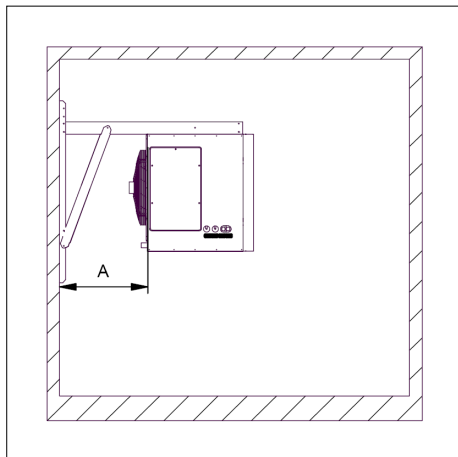
Image 4.2.1.1 : Unité intérieure avec support mural.
