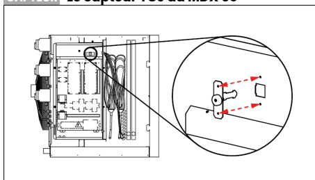
Image 7.5.1.13 : Capteurs TA du Mistral MDX 60.
