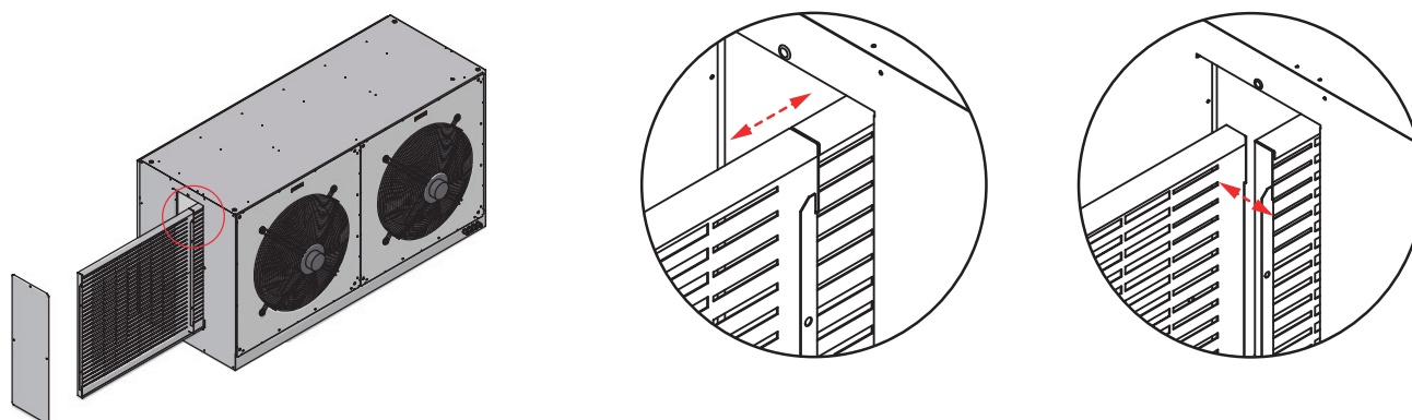
Afbeelding 4.1 Luchtverdeelplaat reinigen
