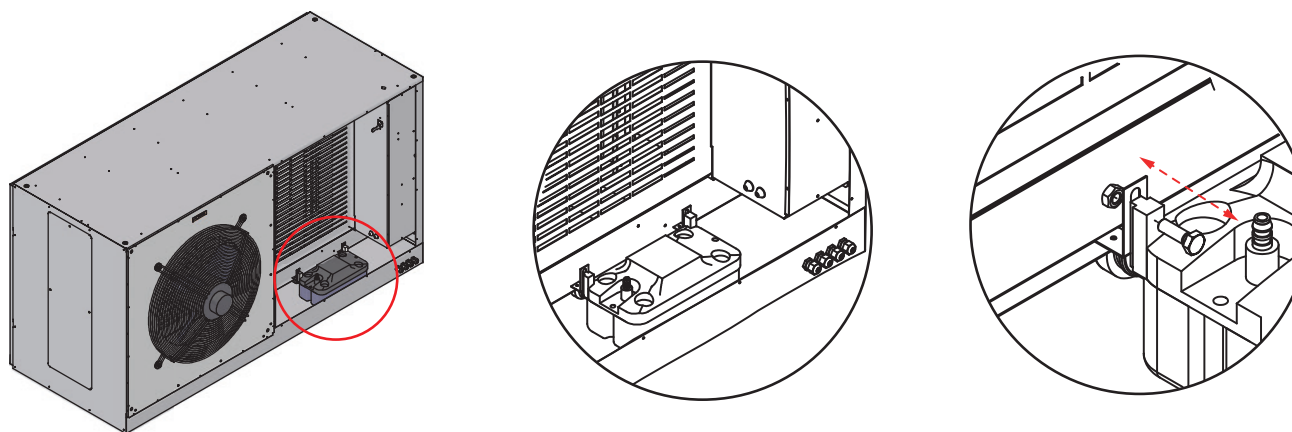
Afbeelding 4.4 Een kapotte condensaatpomp vervangen
